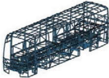
Con la estructura sólida de anillo cerrado, la deformación máxima de la columna solo es de 260 mm en caso de vuelco
