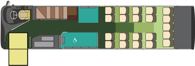
Piso 1: 21 plazas + 6 sillones plegables + 1 silla de conductor
